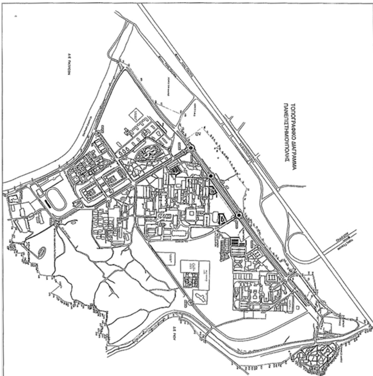
Εικόνα 23. Τοπογραφικό διάγραμμα Πανεπιστημιούπολης
